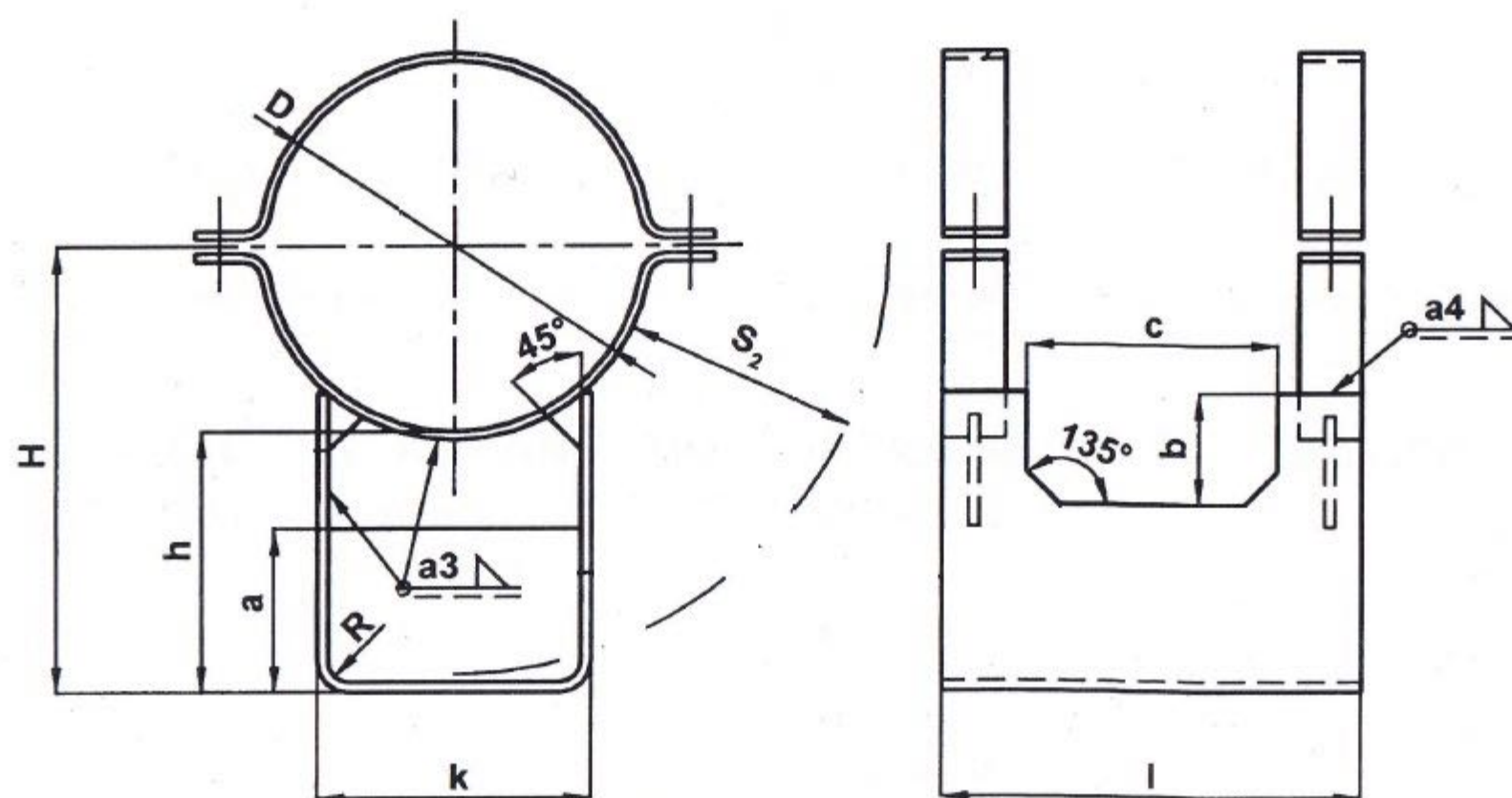
Kuva 1 Liukukannatin Figure 1 Pipe slide
