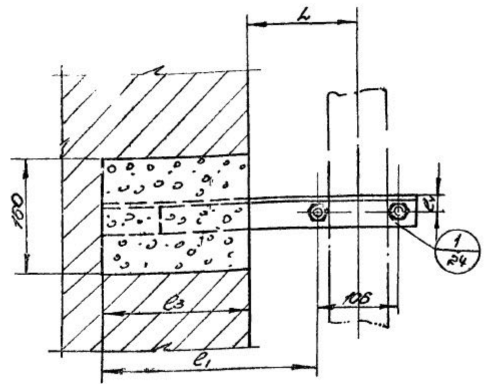
Размеры опор для крепления газопровода с изоляцией. Размеры в мм.
